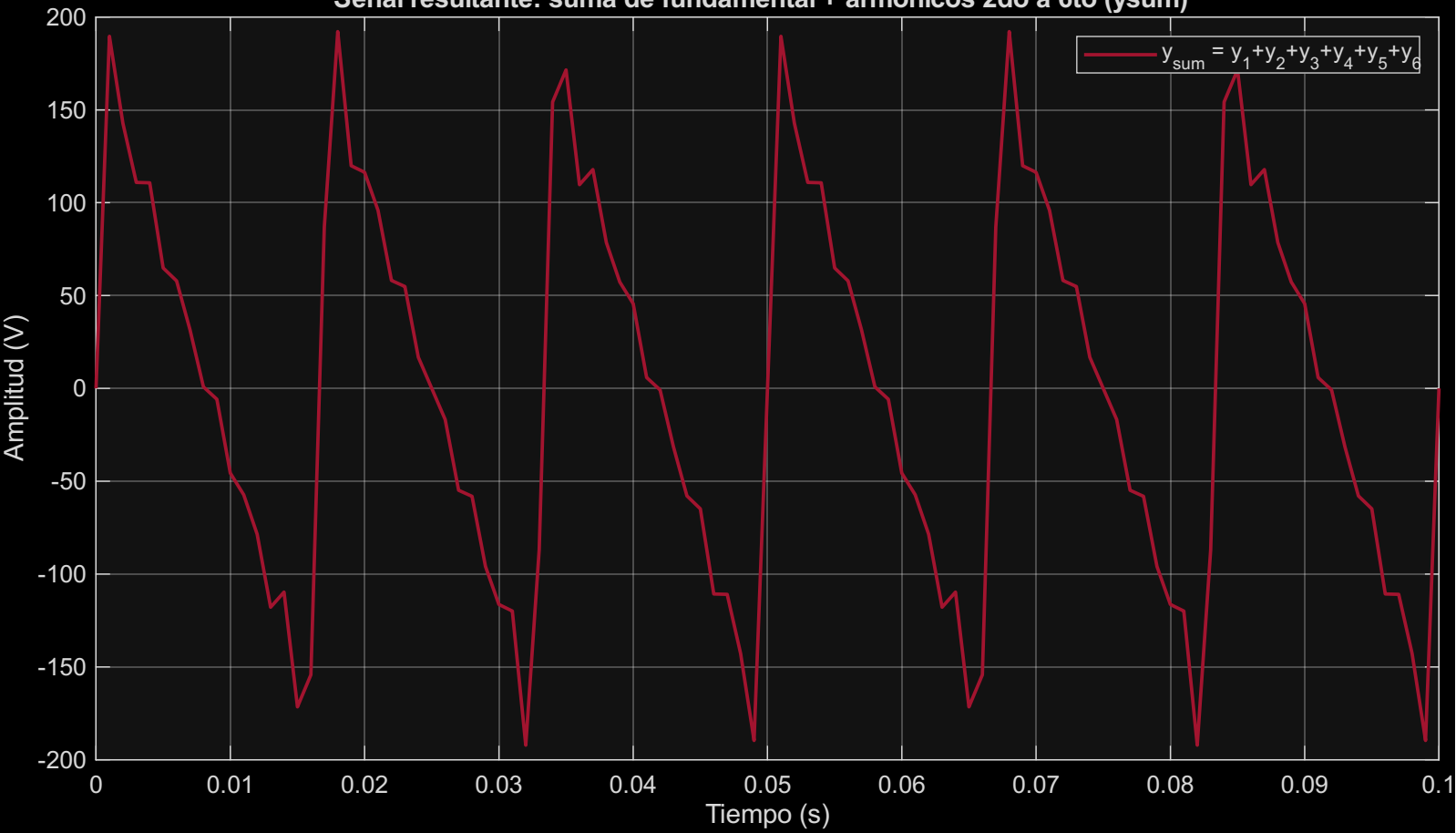
Señal resultante: suma de fundamental + armónicos 2do a 6to (y sum )
